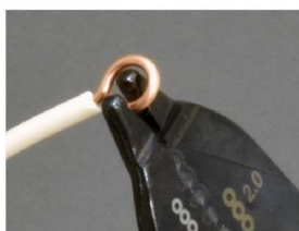
先端で輪作り
