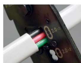
ケーブルをストリッパ
